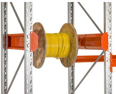
Kabeltrumeloppheeng - med selvåsende aksel. Justerbar fiksering av kabeltrummel samt flyttbar akselplassering i dybden. Seksjonsbredde : 950 og 1350 mm.
