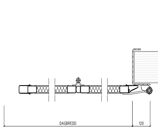
Overmontert motor med arm ved begrenset siderom
