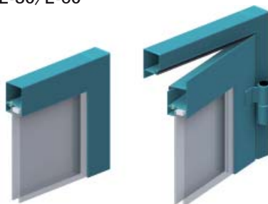
Snitt glasat väggparti
