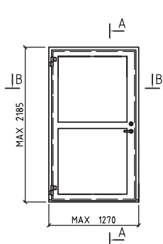
ENKELFLYGLIG SÄKERHETSDÖRR SS-EN 1627:2011 RC 2
