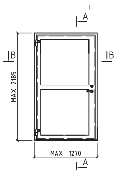
ENKELFLYGLIG SÄKERHETSDÖRR SS-EN 1627:2011 RC 3
