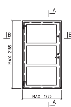
ENKELFLYGLIG SÄKERHETSDÖRR SS-EN 1627:2011 RC 4
