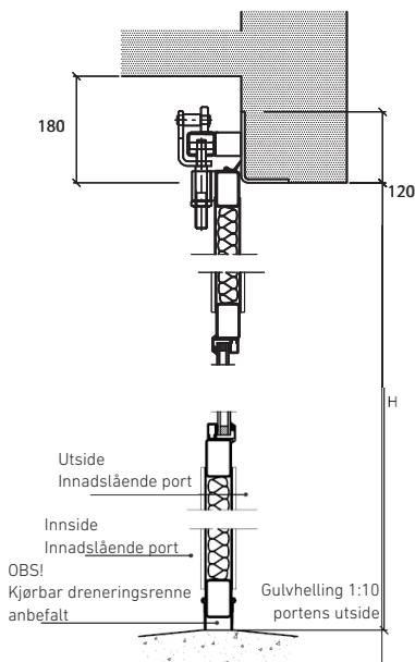
Bæreslag
