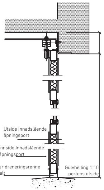
Styrebeslag
