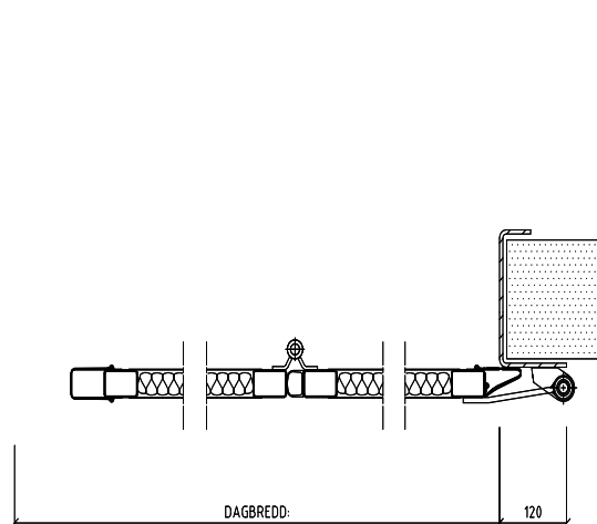
Overmontert motor med arm ved begrenset siderom
