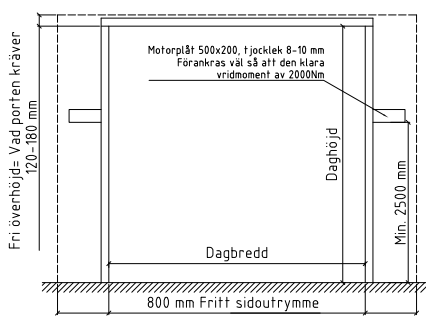
Sidemontert motor
