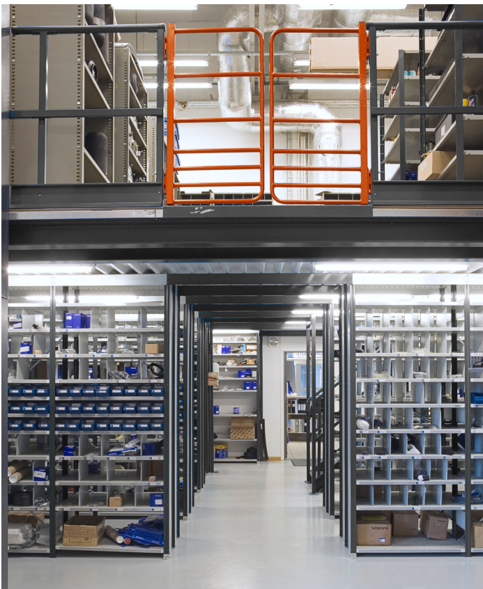
I et plukkager kan mesaninen bygges på EABs hyllereol. Her med opplastingsplass med selvstengende grind.
