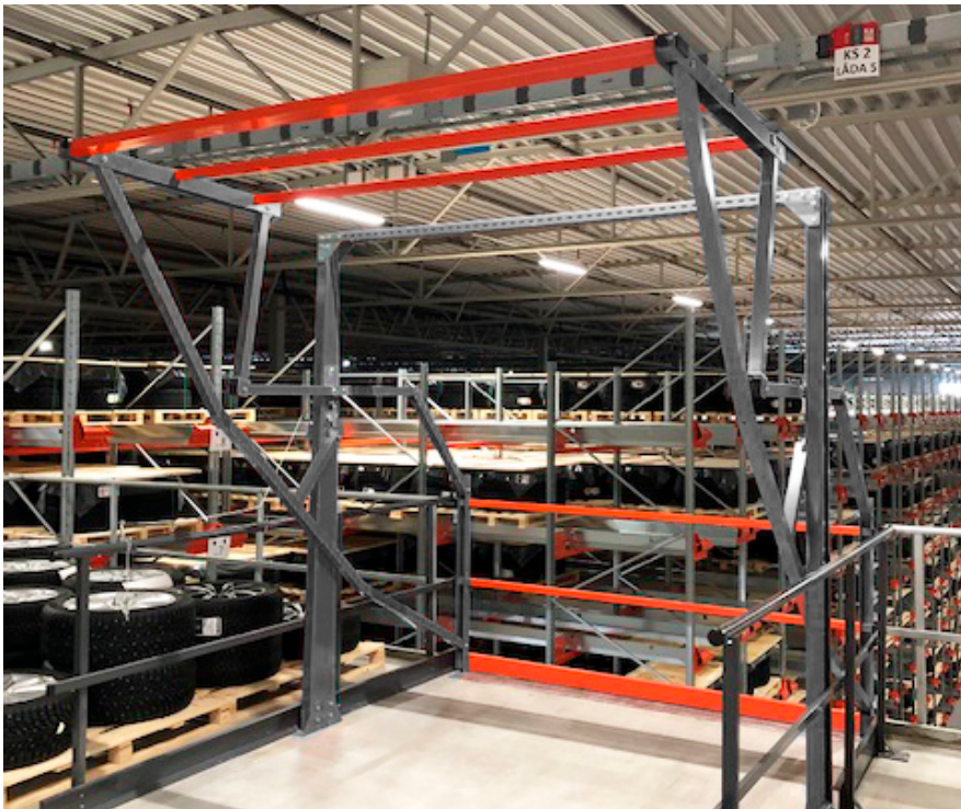
Opplastingsplass med vippegrind
