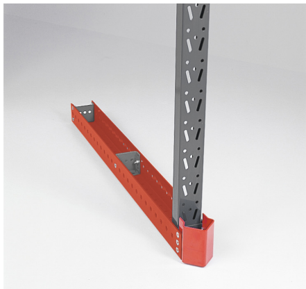
Kraftig bunnprofil med innstyring for trucken.
